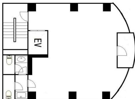
間取り図
